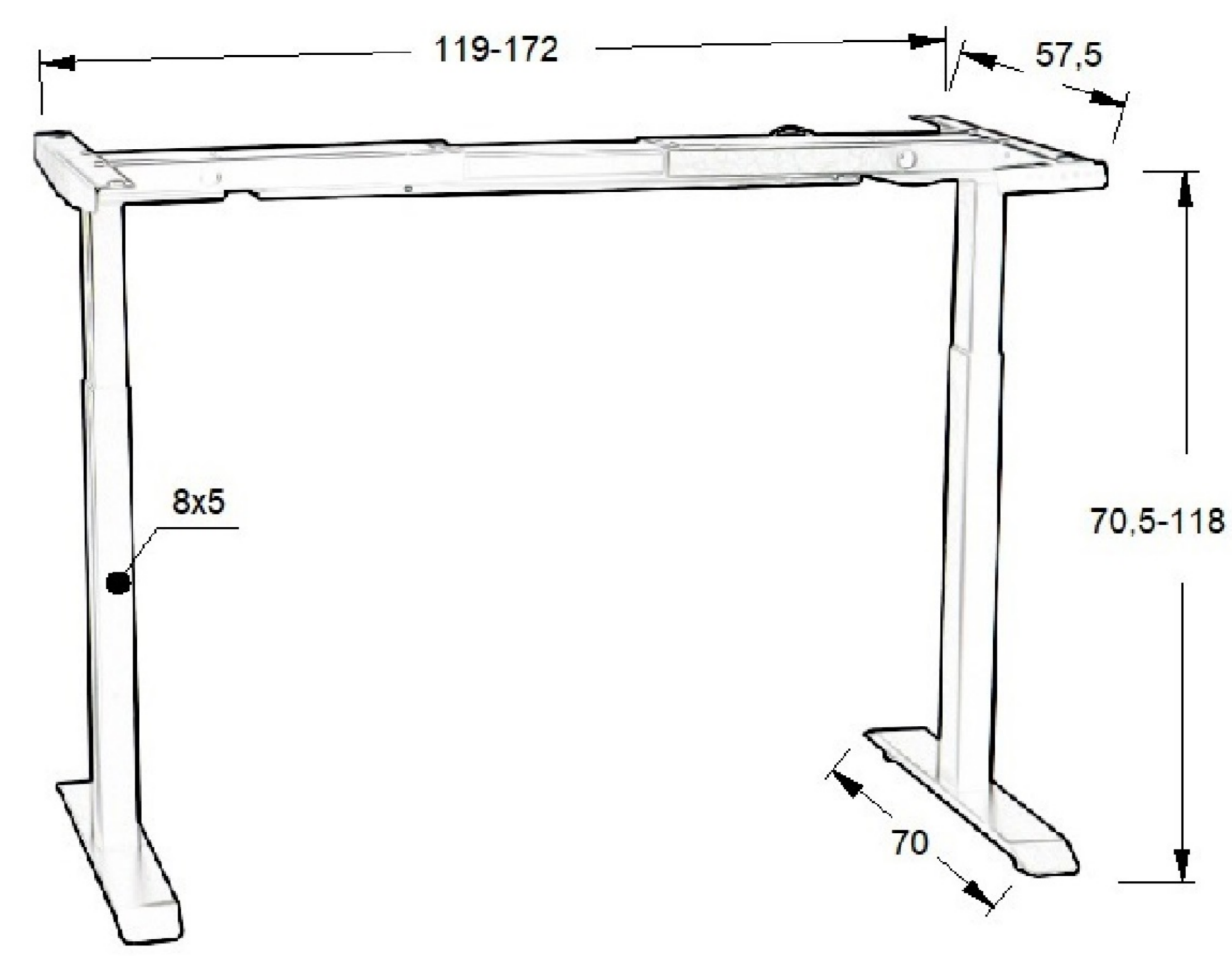
Stelaż elektryczny
